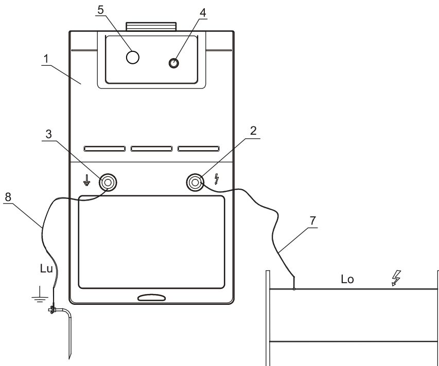
Rys. 2. Części składowe i sposób przyłączenia elektryzatora ECOSTOP 370 do zasilacza AC 12V/150mA, do linii ogrodzenia /Lo/ i do linii uziemienia /Lu/
