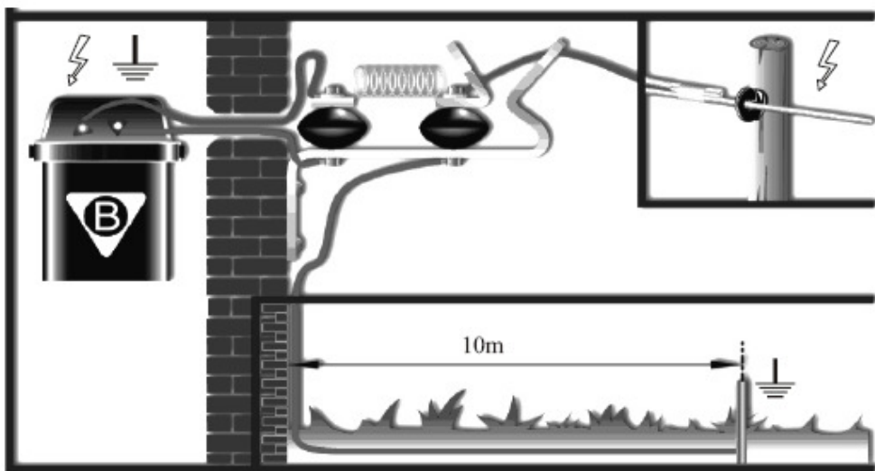
Rys. 5. Sposób przyłączenia odgromnika
