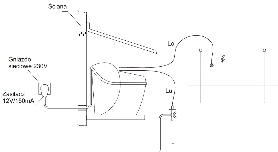
Rys. 4. Sposób instalowania elektryzatora ECOSTOP 370 zasilanego z sieci poprzez zasilacz AC 12V/150mA. /Lu/ - linia uziemienia, /Lo/ - linia ogrodzenia
