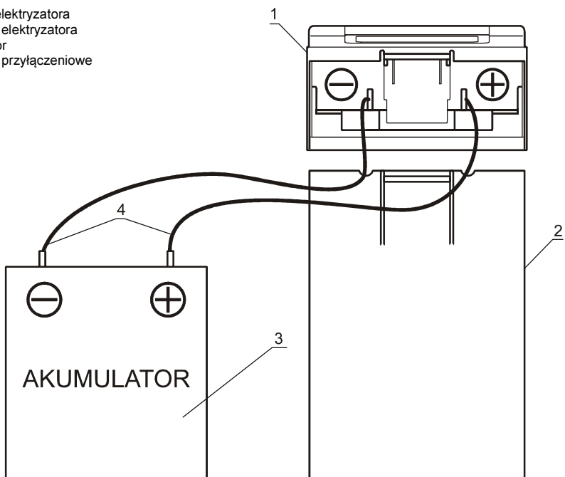
Rys. 3. Sposób przyłączenia elektryzatora ECOSTOP 370 do akumulatora.
